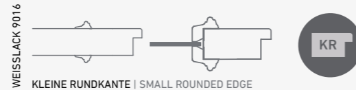
WEISSLACK 9016 KLEINE RUNDKANTE | SMALL ROUNDED EDGE
