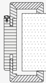
Kleine Rundkante KR1 Small rounded edge KR1
