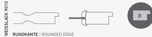
RUNDKANTE | ROUNDED EDGE
